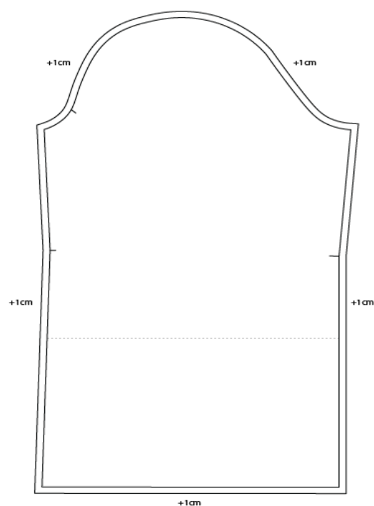
Sl.16 Krojni dio rukava sa šavnim dodacima [27]
