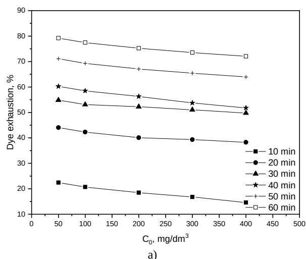
Sl.3 Utjecaj a) koncentracije bojila i b) vremena bojadisanja na stupanj iscrpljenja bojila nakon enzimске hidrolize PET-a
