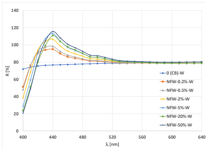
Sl.10 Remisijske krivulje za područje valnih duljina 400-640 nm opranih kemijski i optički bijeljenih pamučnih tkanina s Uvitex NFW različitih koncentracija
