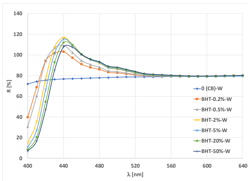
Sl.8 Remisijske krivulje za područje valnih duljina 400-640 nm opranih kemijski i optički bijeljenih pamučnih tkanina s Uvitex BHT različitih koncentracija
