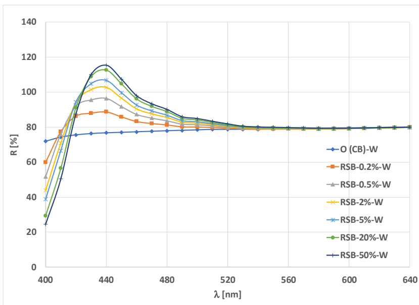
Sl.9 Remisijske krivulje za područje valnih duljina 400-640 nm opranih kemijski i optički bijeljenih pamučnih tkanina s Uvitex RSB različitih koncentracija
