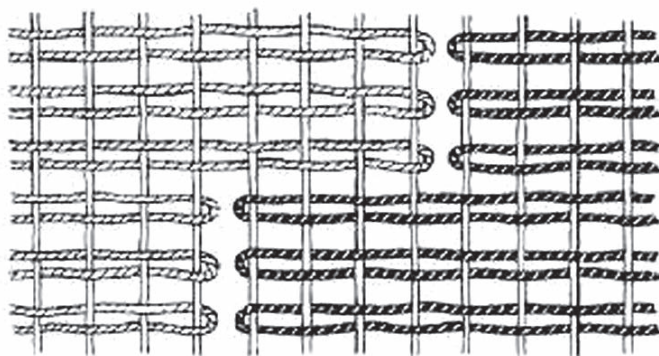
Sl.4 Shematski prikaz Kelem tkanja
