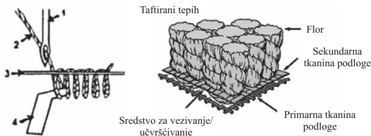
Sl.8 Shematski prikaz tafting postupka
