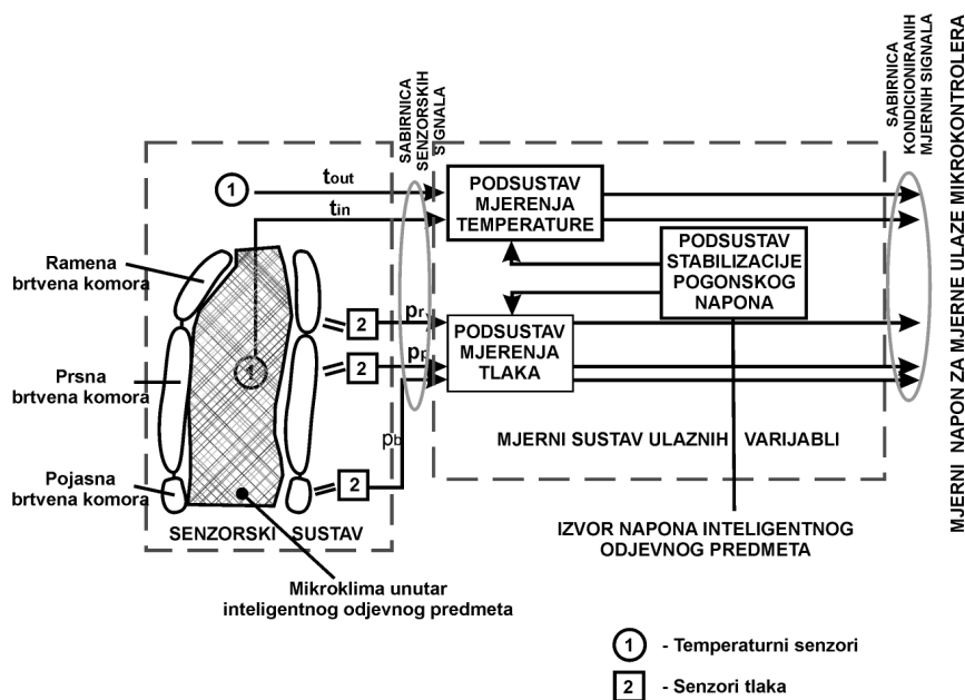
Sl.3 Prikaz senzorskog i mjernog sustava ulaznih varijabli inteligentnog odjevnog predmeta
