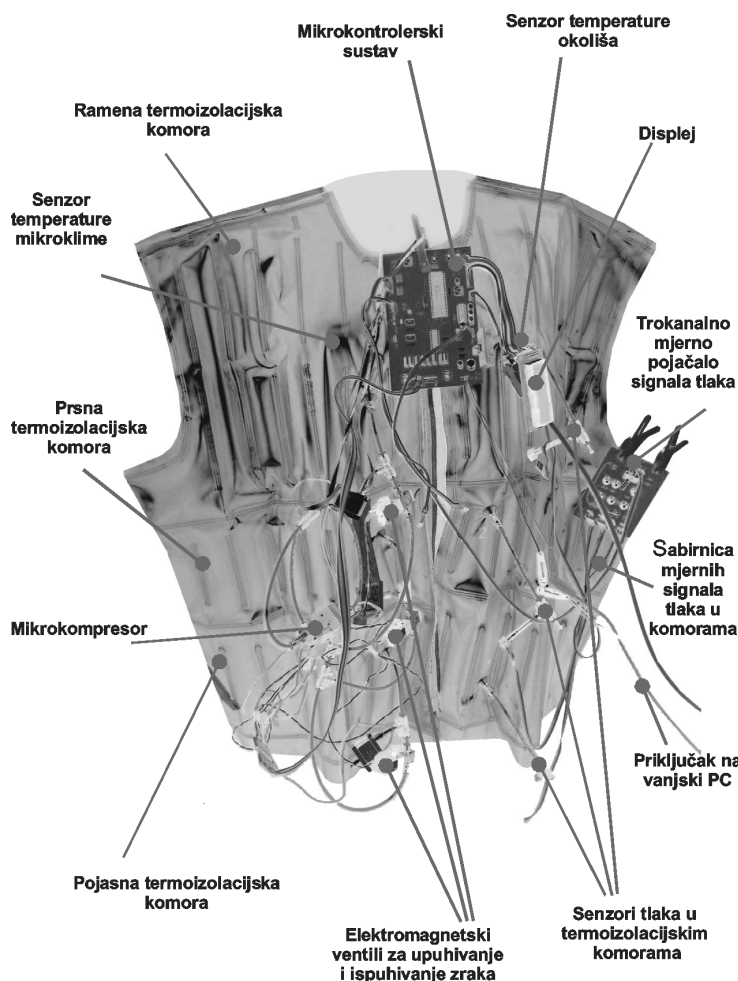
Sl.15 Rezultat završne integracije svih tehničkih podsustava i prva praktična izvedba prototipa prvog inteligentnog odjevnog predmeta s aktivnom termičkom zaštitom
