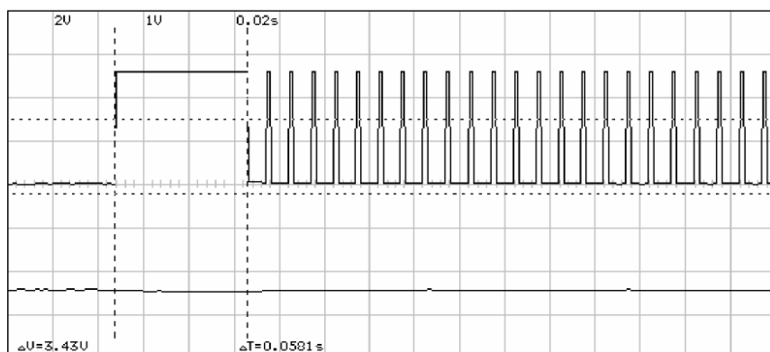
Sl.12 Oscilogram izlaza pomoćnog mikrokontrolera za aktiviranje elektroventila
