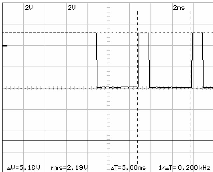
Sl.13 Oscilogram završetka impulsa aktivacije elektroventila punom snagom i prikaz prva dva u nizu PWM impulsa za držanje elektroventila u aktiviranom stanju sa smanjenom snagom aktivacije
