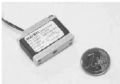
Sl.6 Elektromagnetski ventil oznake 821 2/2 NC, tvrtke Matrix
