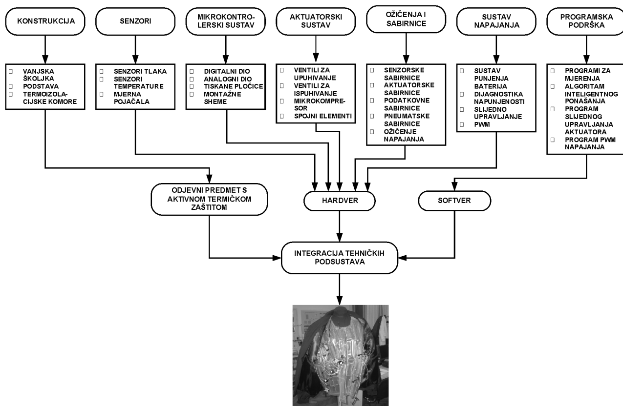
Sl.7 Arhitektura inteligentnog odjevnog predmeta s aktivnom termičkom zaštitom
