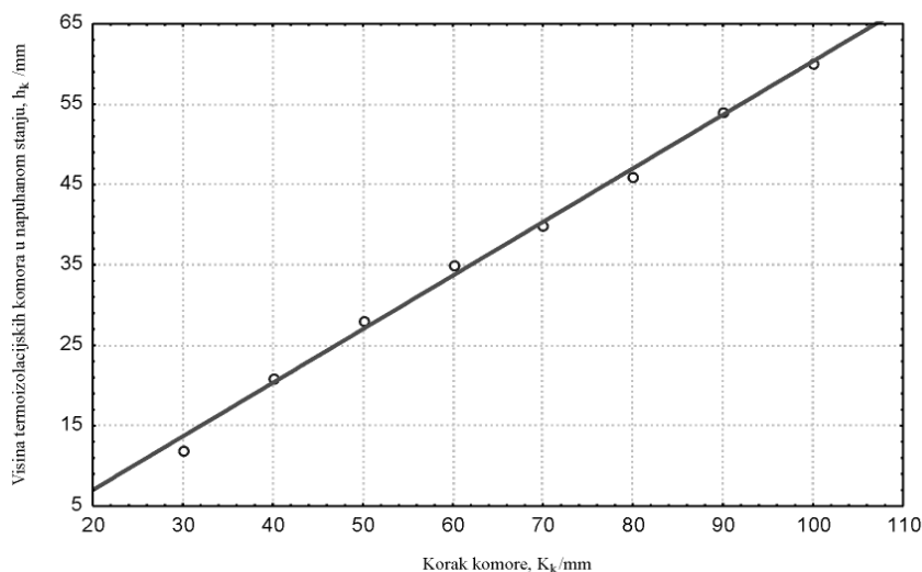
Sl. 10 Ovisnost visina termoizolacijskih komora u napuhanom stanju ( h_k ) pri tlaku od 50 mbar o koracima komora ( K_k )
