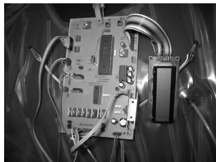
Sl.16 Mikrokontrolerski sustav sa sensorima temperature i displejom
