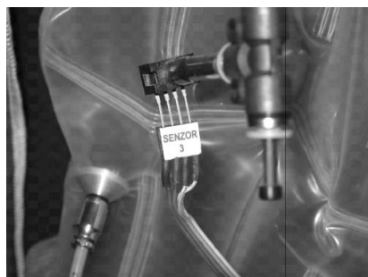
Sl.17 Senzor tlaka ramene komore, priključni konektor i dvodijelni konični priključni element za spoj zrakovoda
